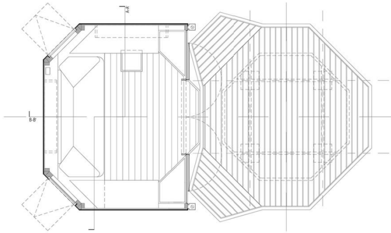
① Planta Poliedro habitable
